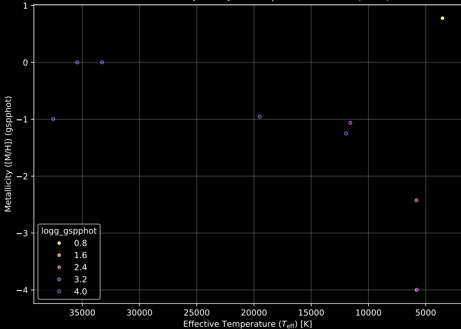
APOGEE DR17 Field: [Bestars] Stellar Population Parameters (n= 10)
